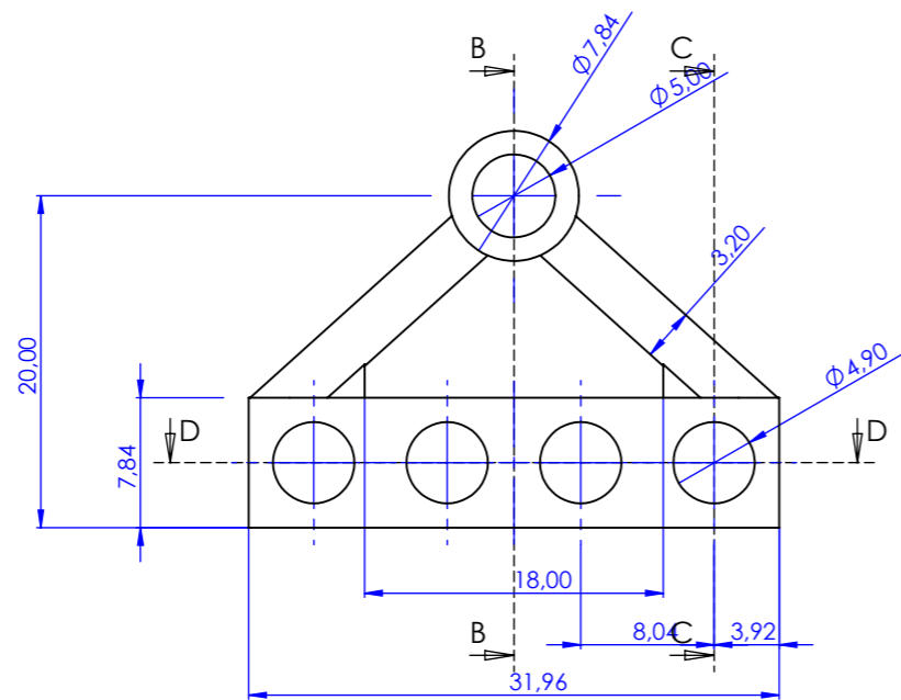
PRZEKRÓJ D-D SKALA 2 : 1
