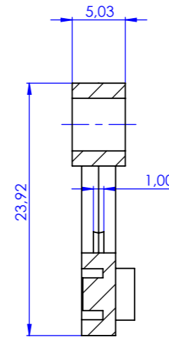
PRZEKRÓJ B-B SKALA 2 : 1
