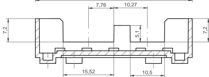
Przekrój C-C
